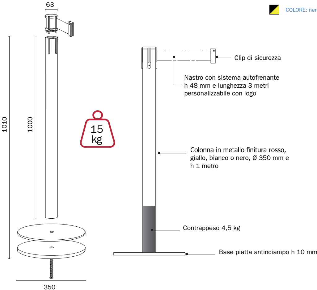
DIMENSIONI PRODOTTO (mm)
