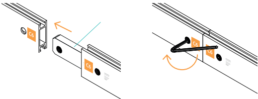
3 Assemblaggio di una traversa ad una cornice
