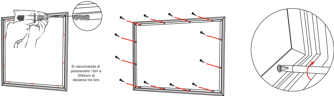
6 Assemblaggio della grafica con bordino in silicone
